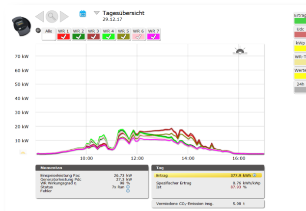
Bild 1: Vergleich einzelner Stränge und Wechselrichter
